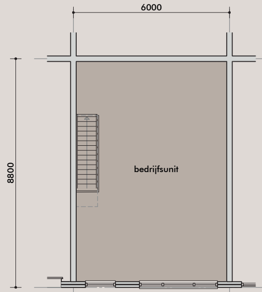
1 e verdieping 52,8 m 2
