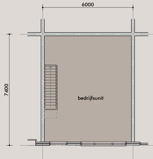
1e verdieping 44,4 m 2
