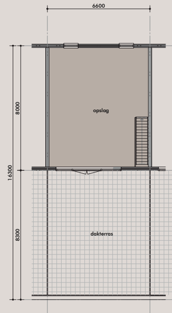
2e verdieping 52,8 m 2
