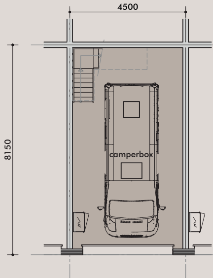
Begane grond 36,7 m 2
