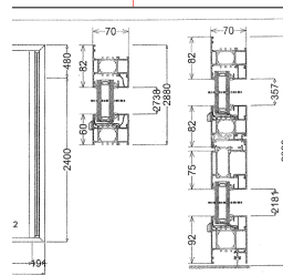
vertikale detail
